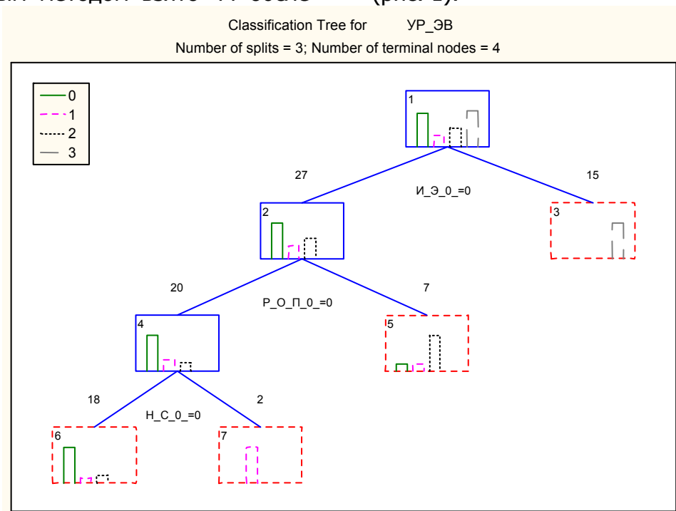
Рис 1. Дерево классификации 1
